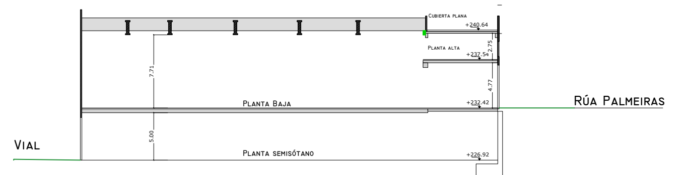
SECCIÓN - E. 1:400
